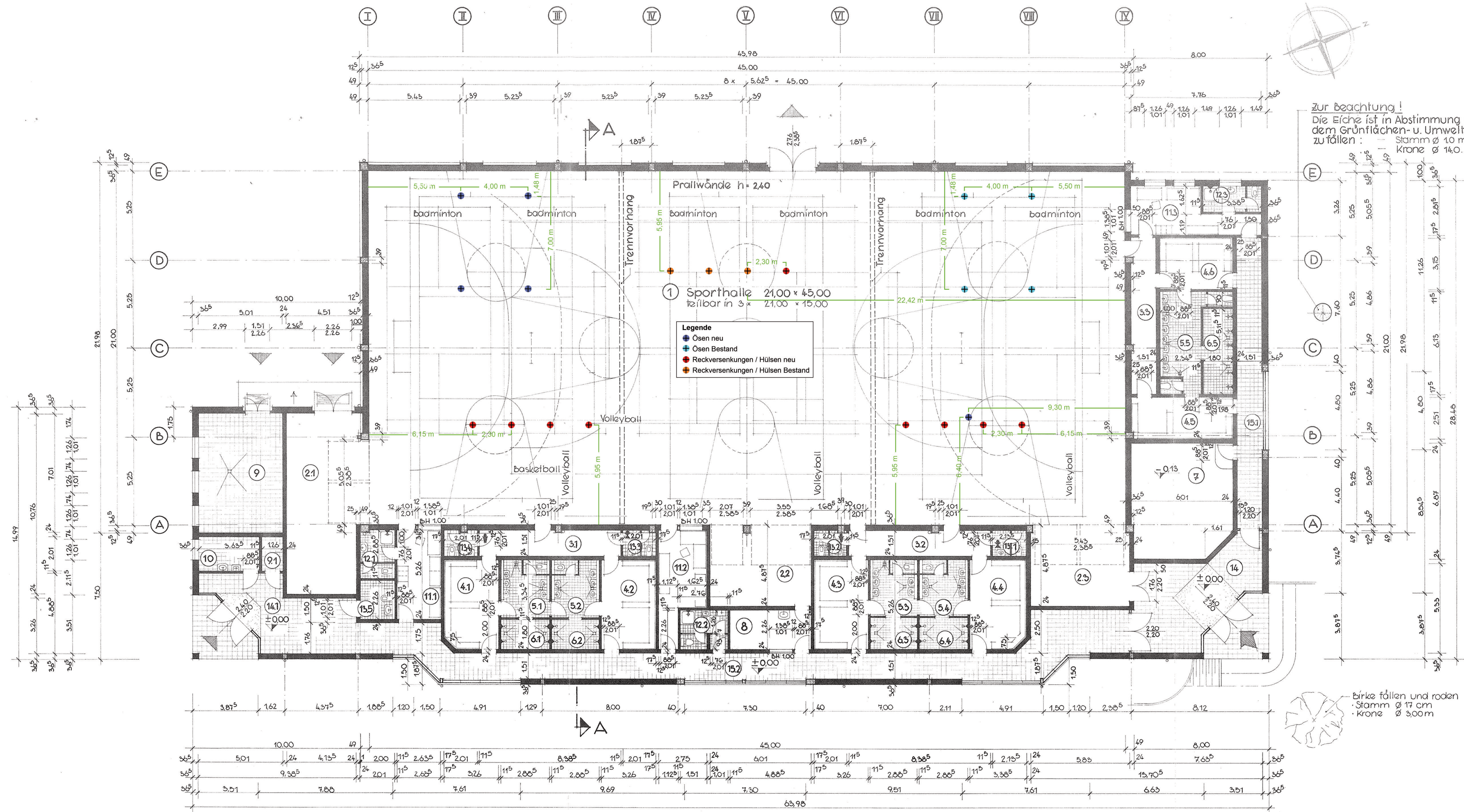
Grundriß M. 1 : 100
